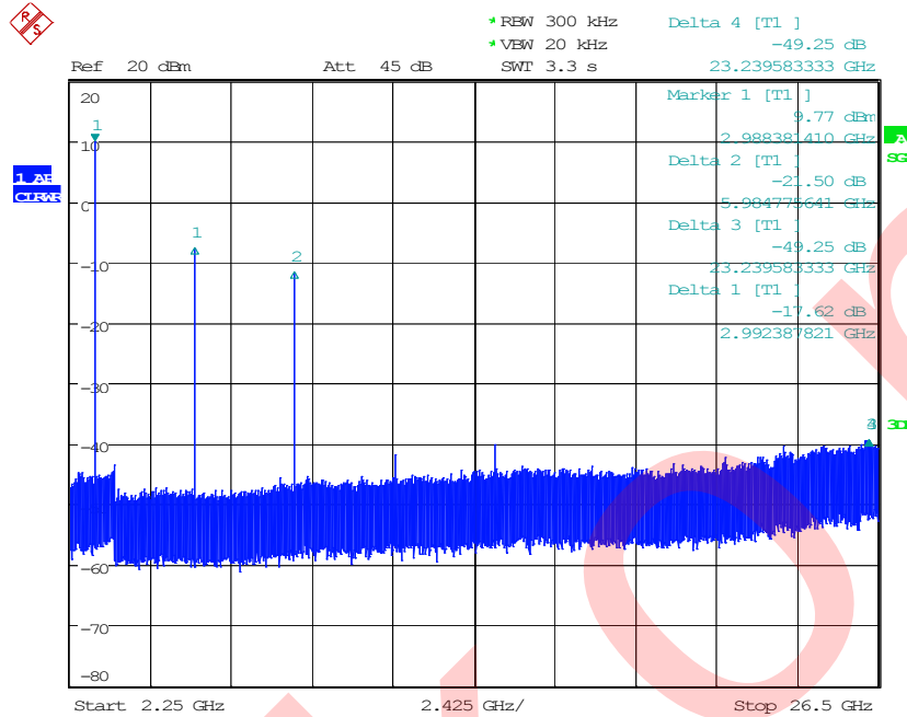
HARMONIC SUPPRESSION
