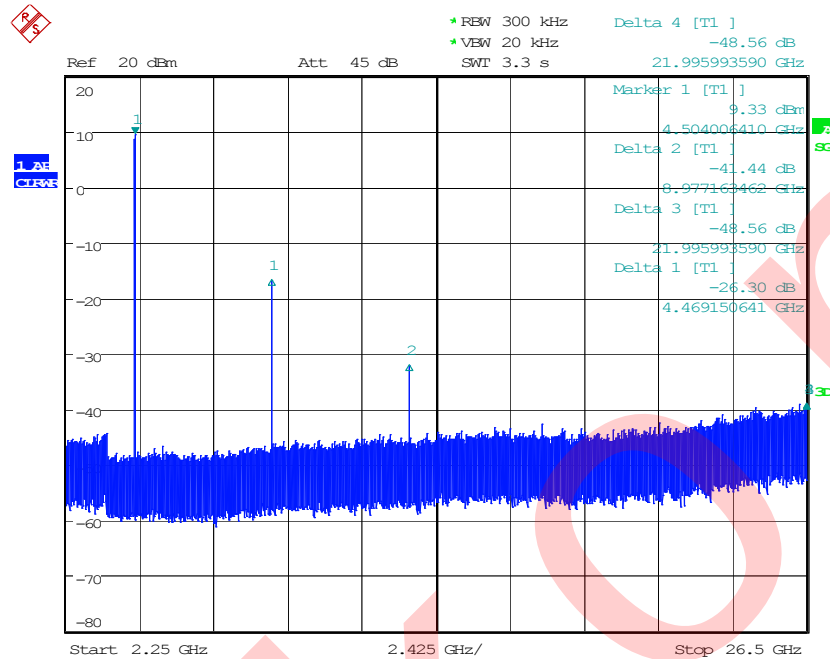
HARMONIC SUPPRESSION
