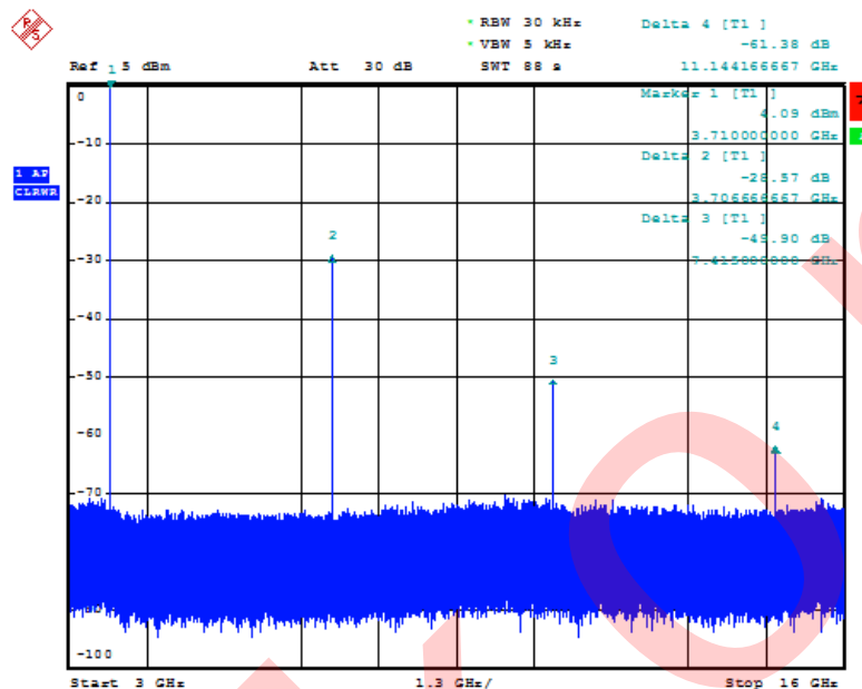
HARMONIC SUPPRESSION
